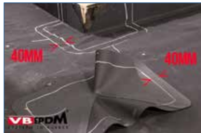
Bild 70. Kleberfreie Bereiche.
